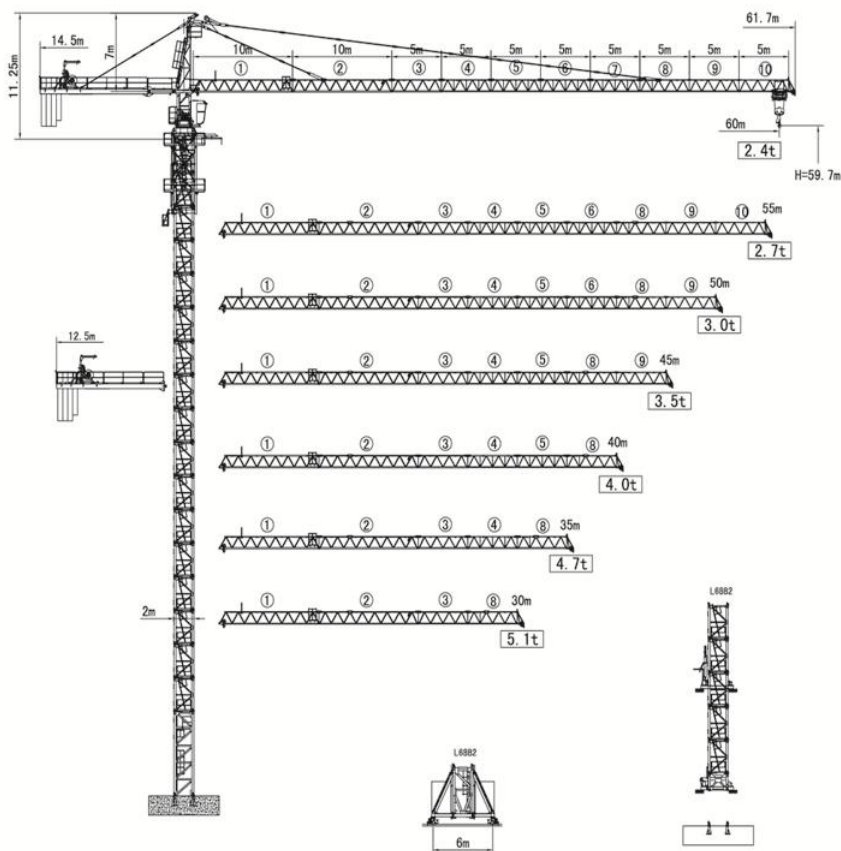
载荷特性表 Load Diagrams 10t
